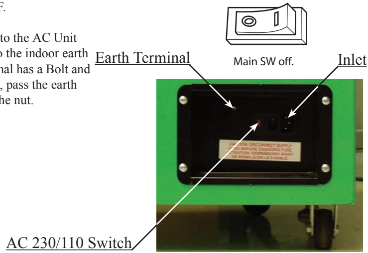
FIG. 6.2a AC Unit
